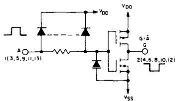
等価回路
